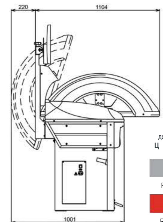
Габаритные размеры СБ
