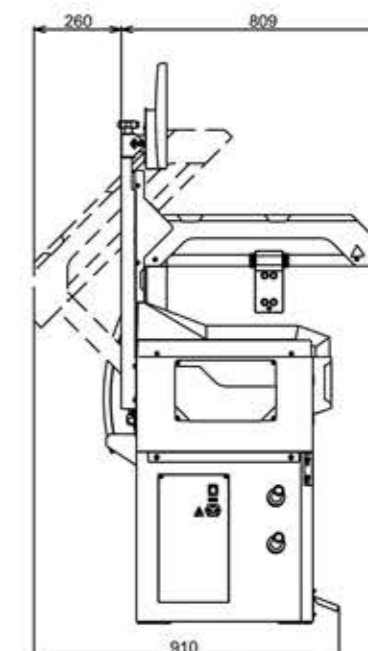
Габаритные размеры СБ
